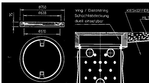
Schachtabdeckung, rund, LW 600, Klasse A 15, Art.Nr. 200-2022 EDV-Bestell-Nr. 85113 Adapter-Ring für Betonringe mit integriertem Deckel
