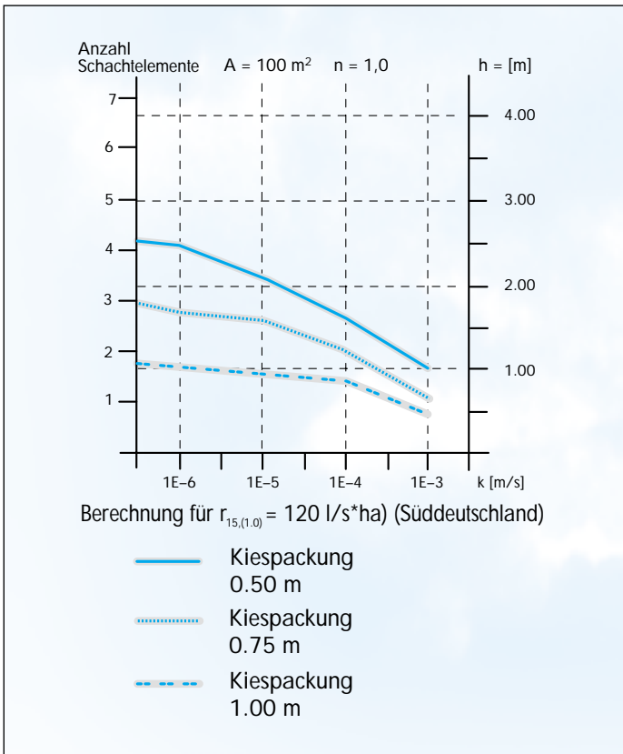
Einfluß der Kiespackung n = 1, = a^{-1}
