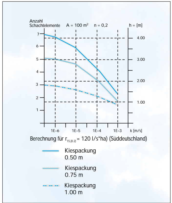
Einfluß der Kiespackung n = 0,2 a^{-1}
