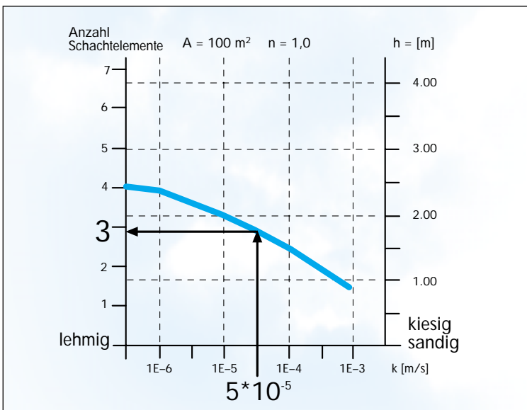
Berechnungsformel und Beispiel zur Ermittlung der Elementanzahl
